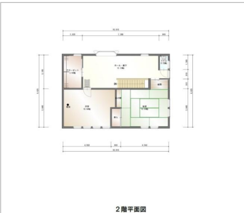
2階平面図
